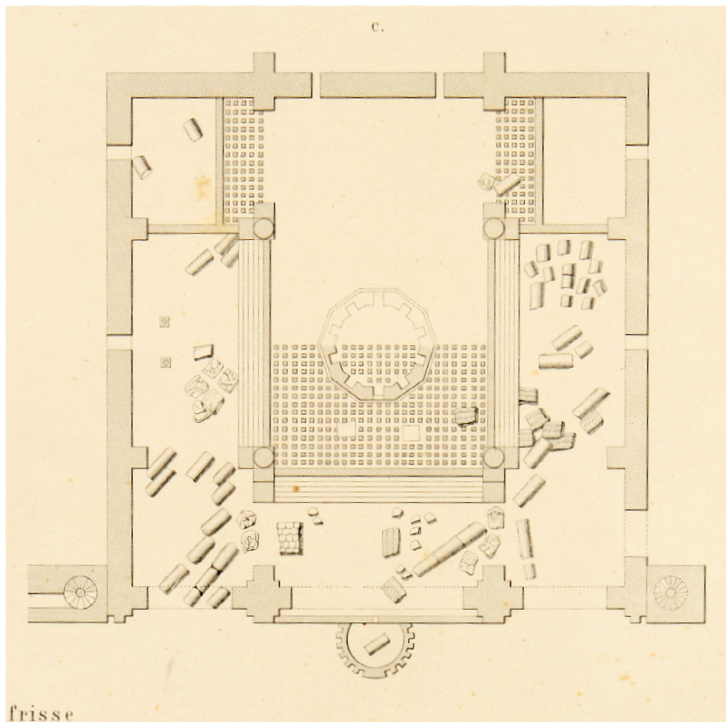
Abb. 3: Zeichnung mit Befunden des Dombrandes im 5. Jahrhundert. Lithographie von Johann Nikolaus von Wilmowsky (1874), Museum am Dom Trier. Foto: Museum am Dom Trier.
