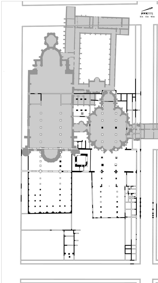
Abb. 2: Grundriss der Trierer Kirchenanlage um 340, Zeichnung A. Hill, Museum am Dom, Trier. Aus: Weber 2022, Abb. 2.
