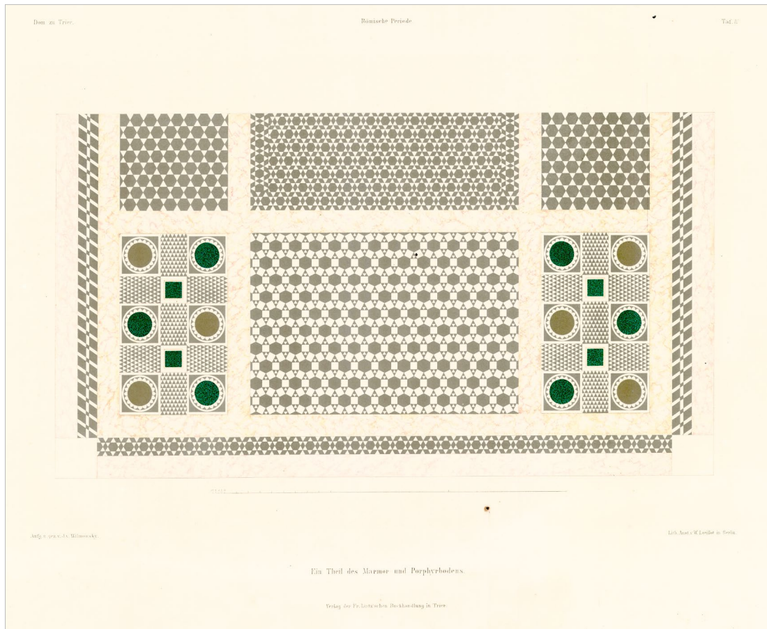
Abb. 4: Rekonstruktionszeichnung des Fußbodenbelags im römischen Kernbau des Trierer Domes. Lithographie von Johann Nikolaus von Wilmowsky (1874), Museum am Dom Trier. Foto: Museum am Dom Trier.
